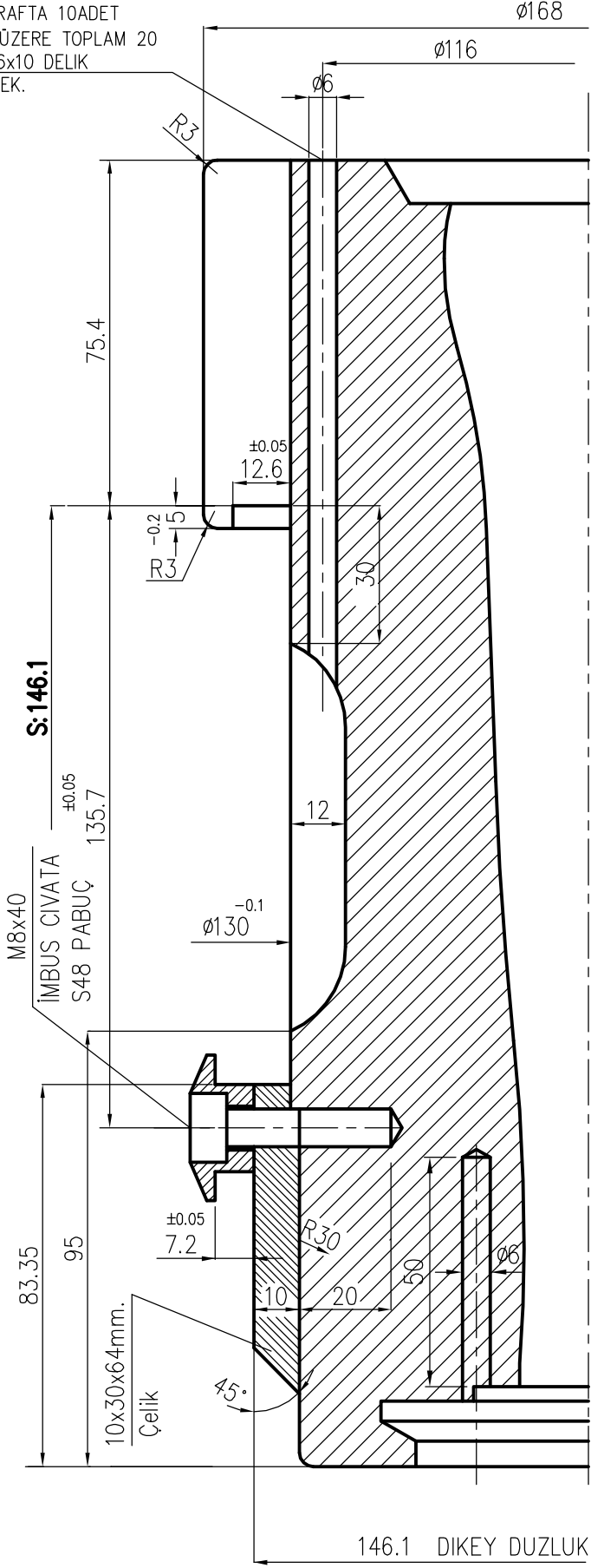
A-A KESİTİ
